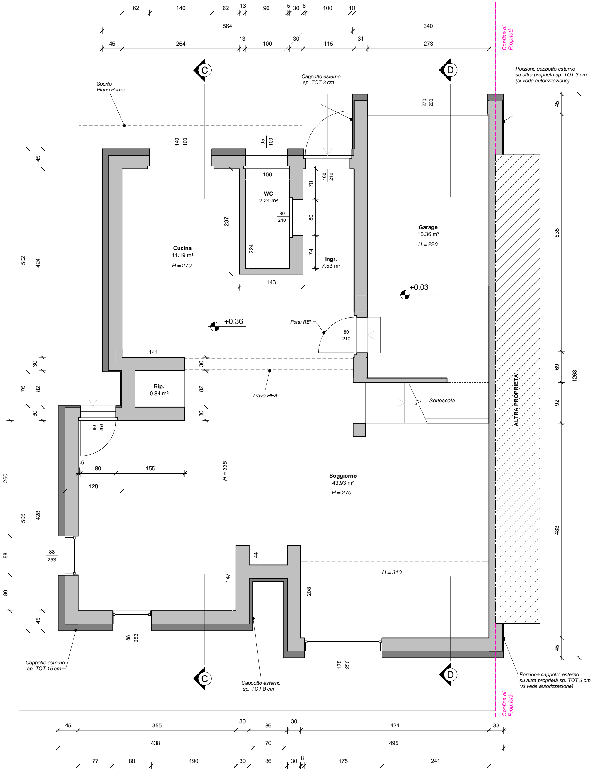
1 Pianta Piano Terra - Progetto Scala 1 : 50
