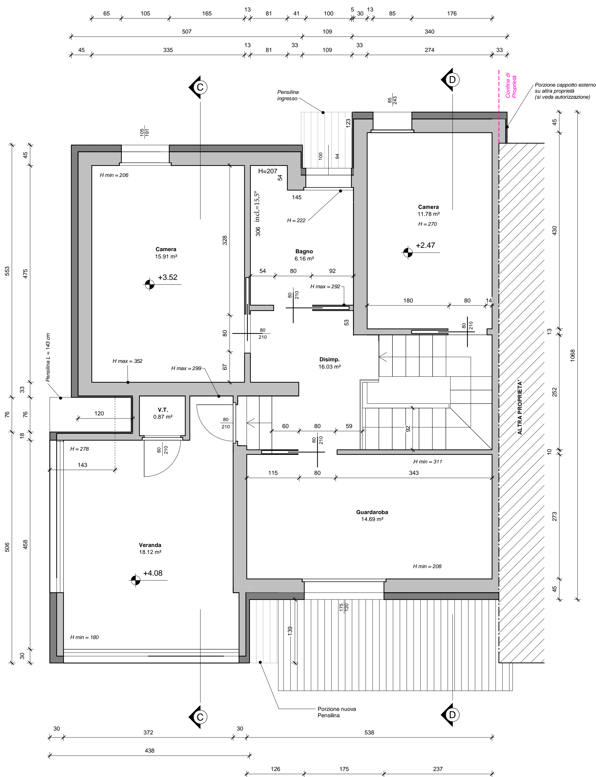
1 Pianta Piano Primo - Progetto Scala 1 : 50
